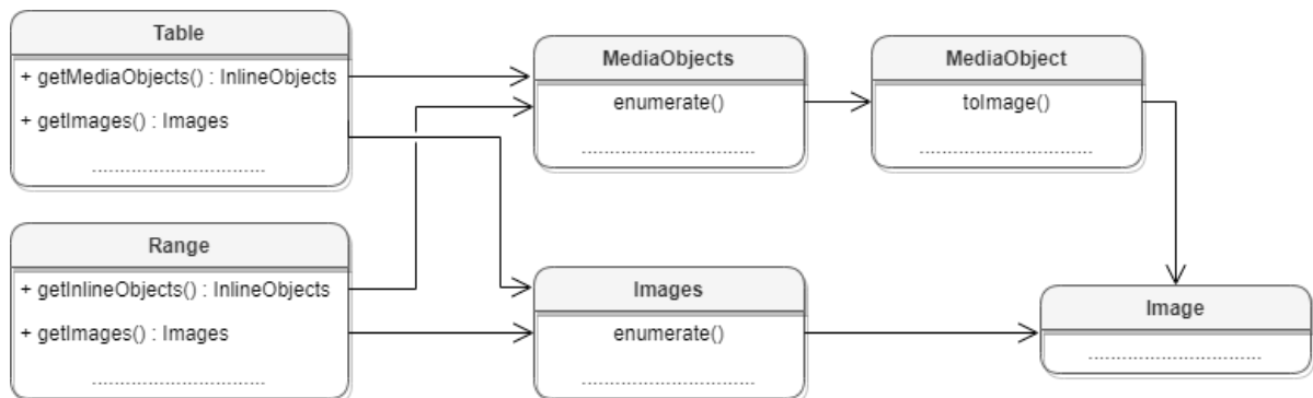
Рисунок 32 – Графические объекты
