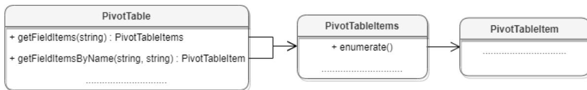
Рисунок 39 – Объектная модель таблиц для работы с элементами сводных таблиц
