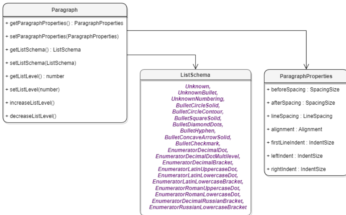
Рисунок 33 – Объектная модель таблиц для работы со свойствами параграфа
