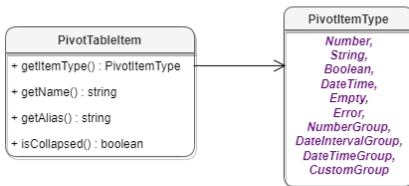
Рисунок 38 – Таблица DocumentAPI.PivotTableItem
